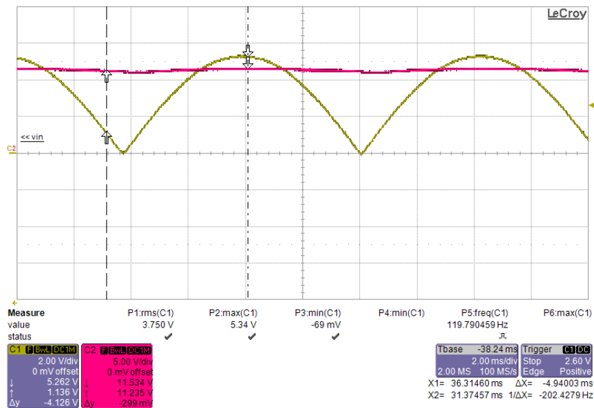
Fig-8. Phase_In & 68nF & SOURCE
