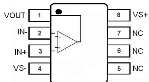
TSSOP-8
