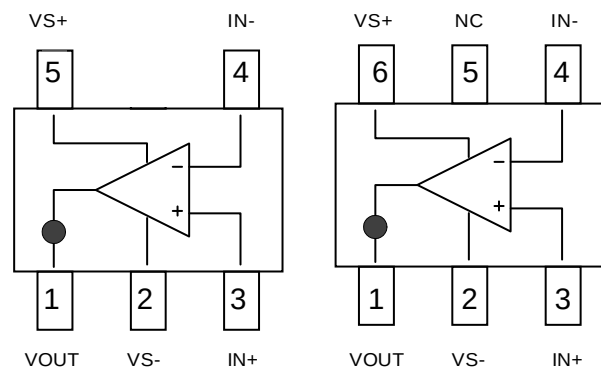
SOT25/TSOT25
