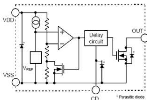
OPEN DRAIN ( EC9508C )
