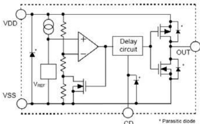
CMOS OUTPUT ( EC9509C )
