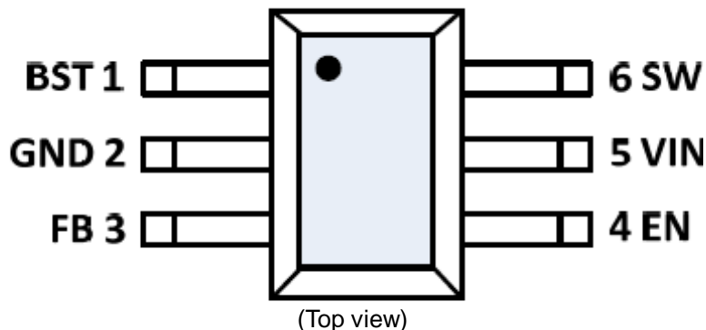
SOT23-6
