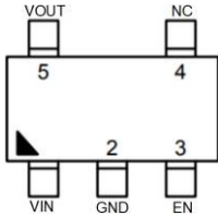
SOT-23-5
